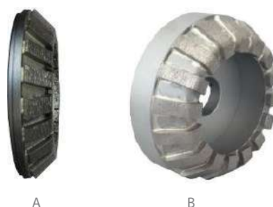
PRECUT WHEEL MOLA PRE-TAGLIO
